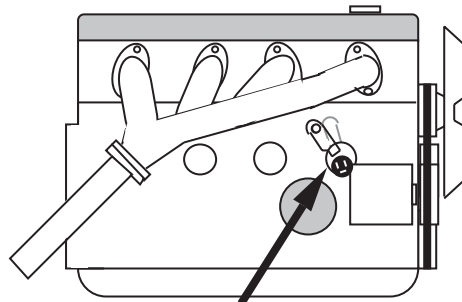
VOLVO 240 1991-1992 : ⚙B200 • ⚙B230F
